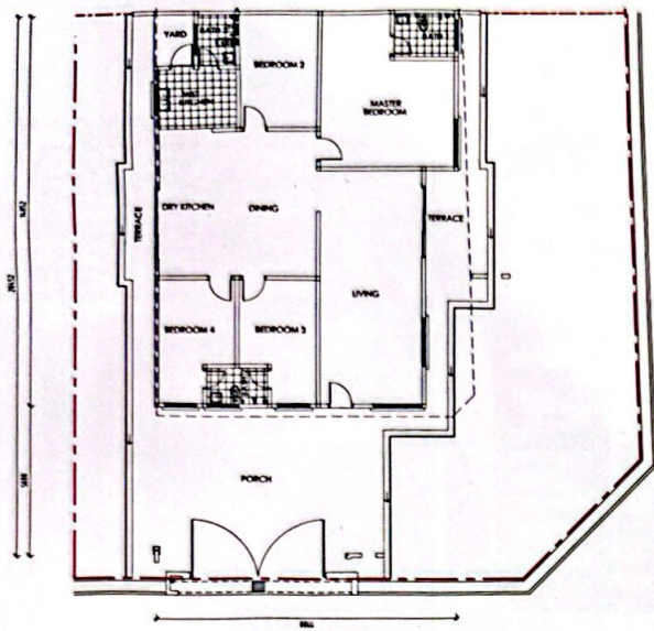
Rumah Berkembar Setingkat (Jenis A)
