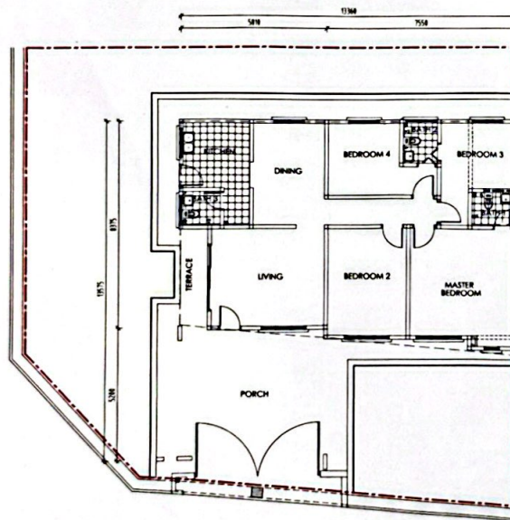
Rumah Berkembar Setingkat (Jenis C)
