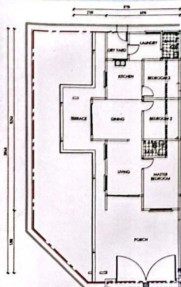
Rumah Teres Setingkat (Jenis A)
