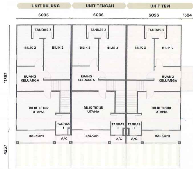
Aras Atas
